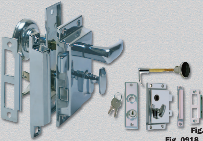
Fig. 0918/0919 Shown Assembled
